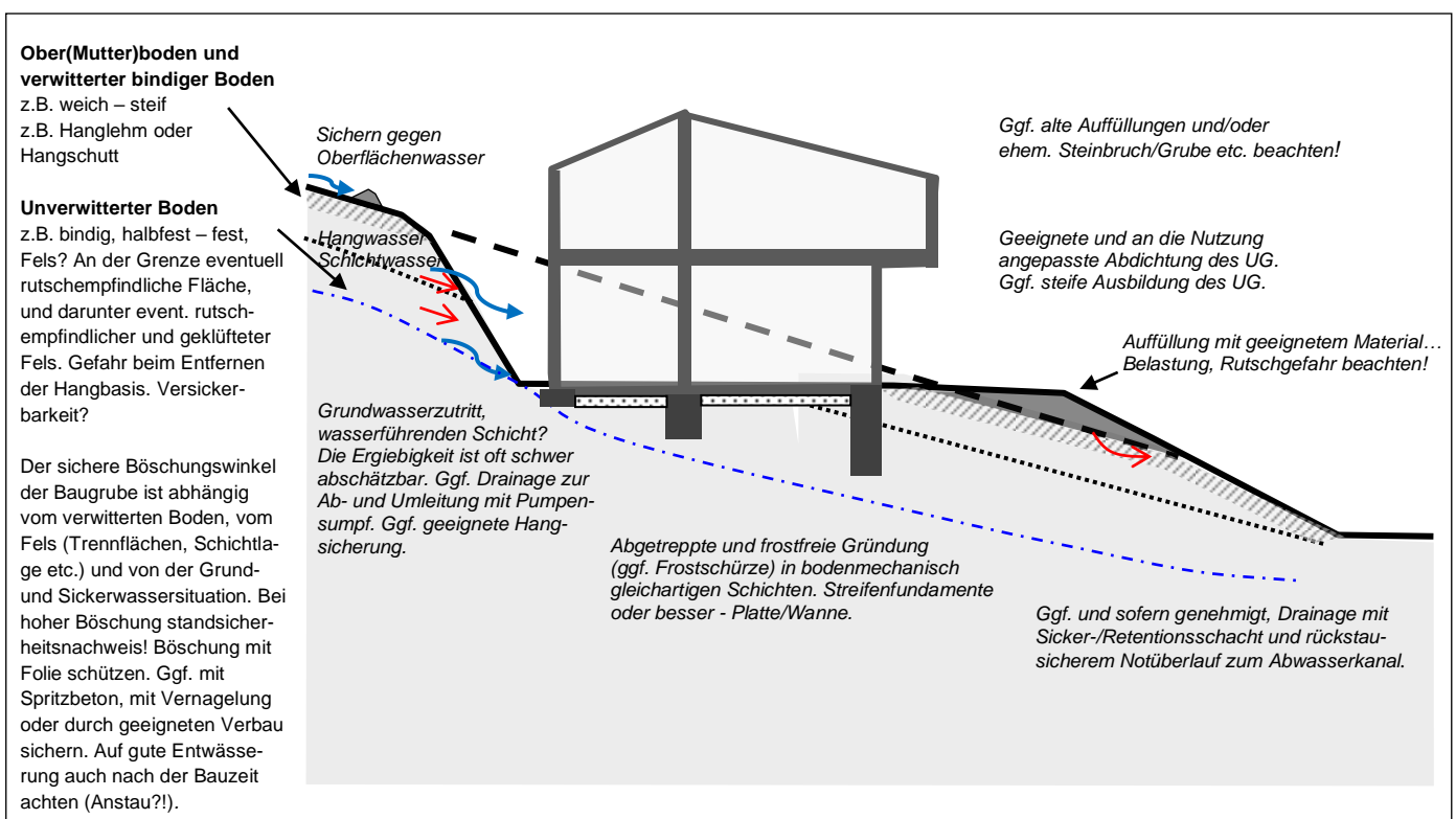
Abb. 18: Bauen am Hang (schematisches Beispiel)
