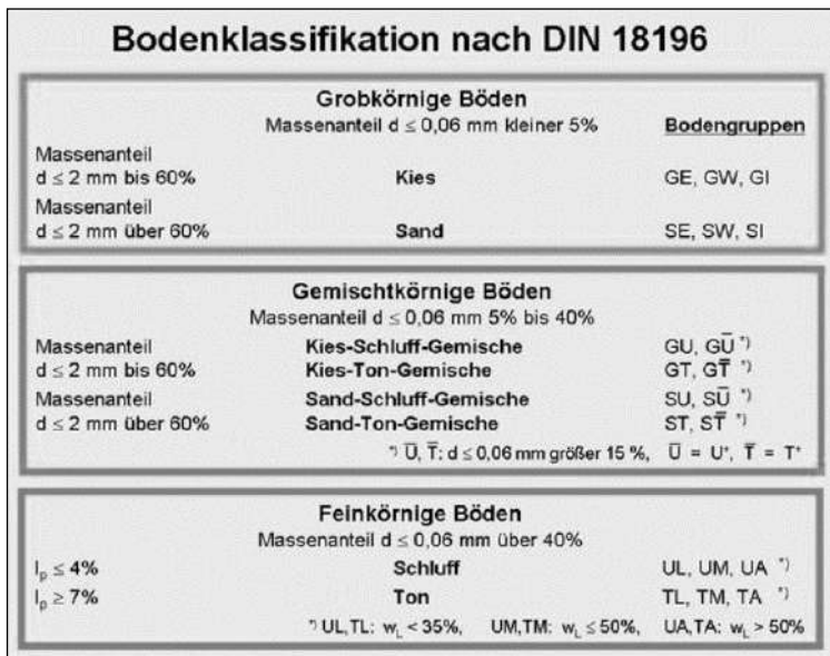
Abb.12: Bodenklassifikation nach DIN 18196. Grafik aus: Bodenmechanisches Praktikum, HS Bielefeld - Labor für Bodenmechanik, Prof. Dr.-Ing. Antje Müller-Kirchenbauer, Dipl. Ing. (FH) Holger Paetsch. Abkürzungen der Bodengruppen siehe Tabelle 7, 8e. Querstrich = stark
