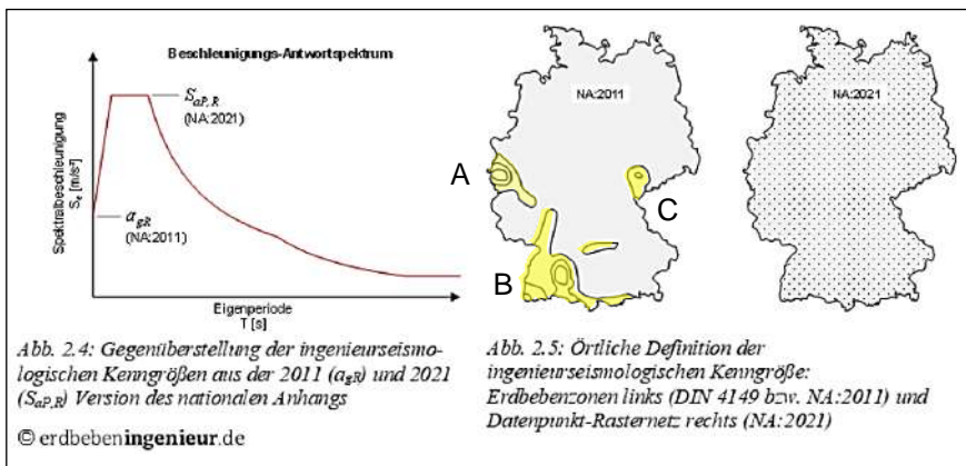
Abb. 9a: Vergleich ingenieurseismische Kenngrößen - alte DIN 4149 – NA 2011, neue DIN EN 1998-1:2010-12, NA 2021. Quelle ergänzt: Dipl.-Ing. Marius Pinkawa, https://erdbebeningenieur.de/
