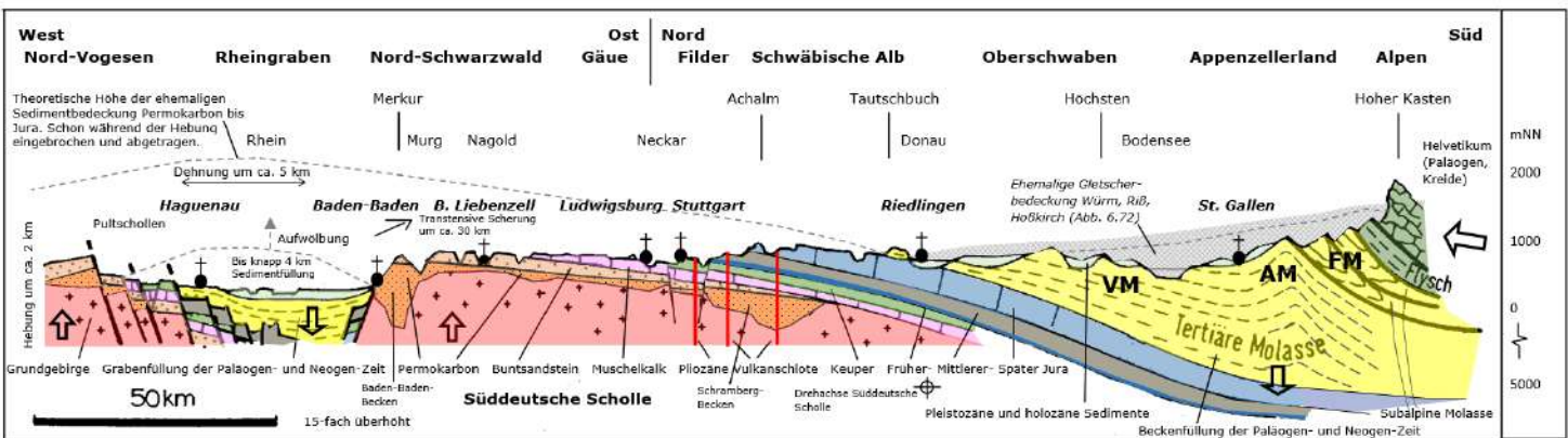
Abb. 2: Geologischer Profilschnitt von Baden-Württemberg - schematisch und ca. 15-fach überhöht. Die geologische Karte und der Profilschnitt verdeutlichen den dreidimensionalen Aufbau des Untergrundes. Die Pfeile zeigen die relativen Hebungen und Absenkungen und den Schub durch die Alpenbildung. VM = Vorlandmolasse, AM = Aufgerichtete Vorlandmolasse, FM = Faltenmolasse. Die Sedimentbedeckung über Rheingraben, Schwarzwald und Schichtstufenland wird seit etwa 145 Mio. Jahren abgetragen. Grafik verändert und ergänzt nach: O. F. Geyer & M. P. Gwinner (1991), Geologie von Baden-Württemberg.
