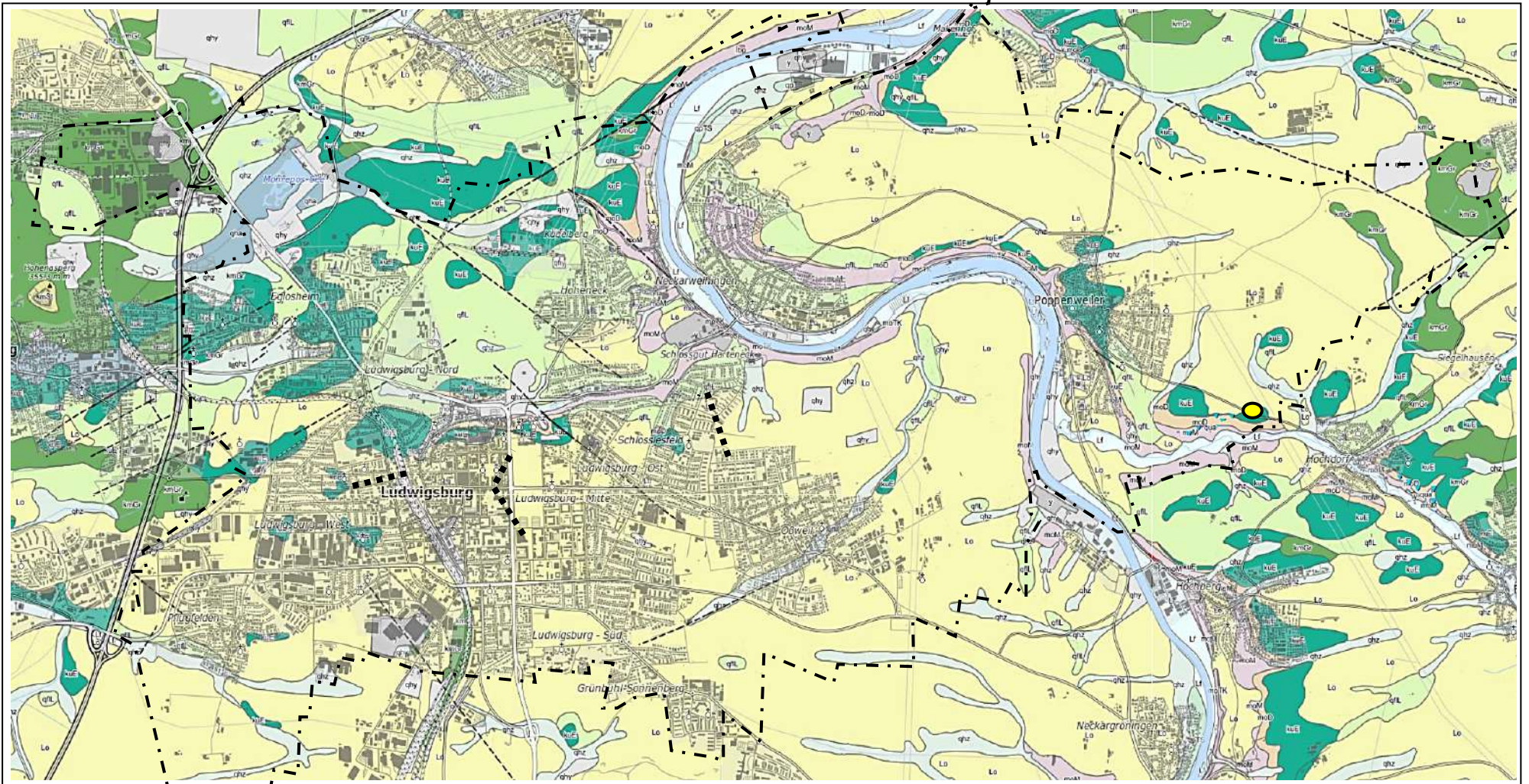
Abb. 5a: Geologische Karte von Ludwigburg.
