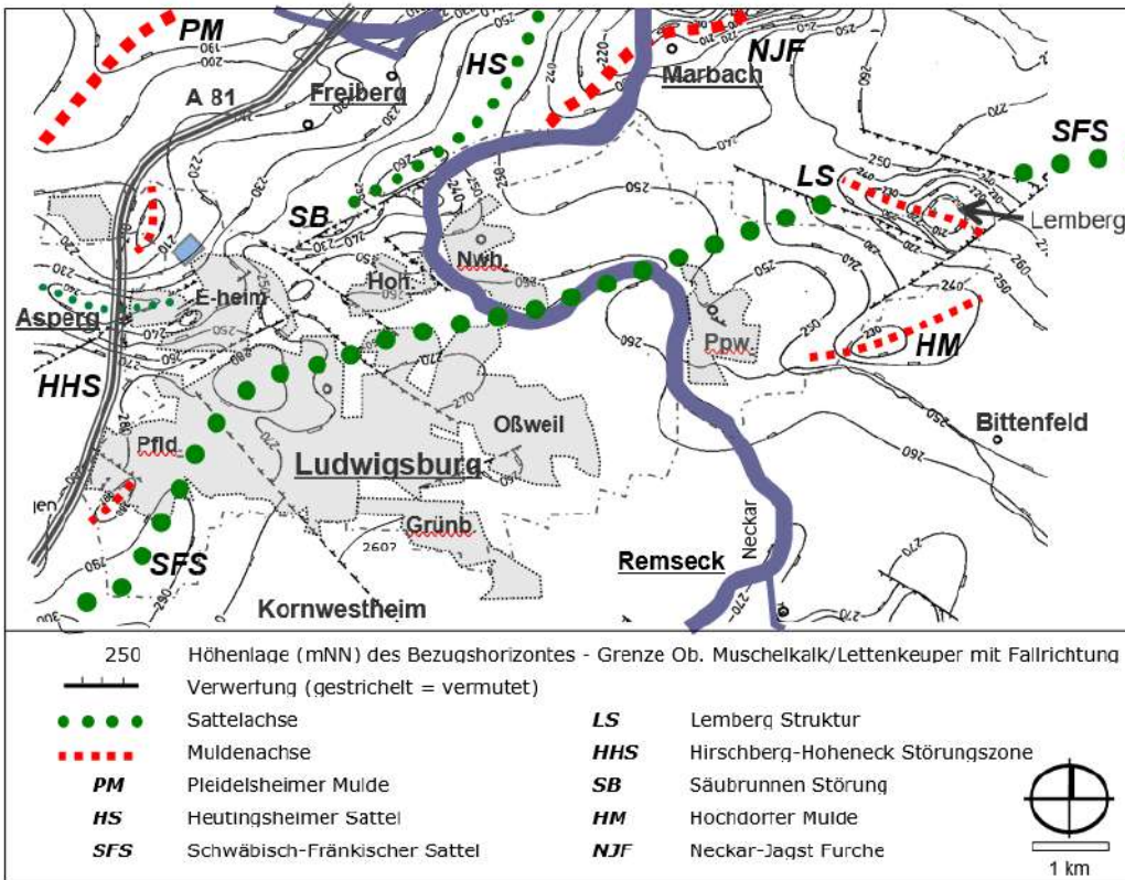
Abb. 8: Schichtlagerung und tektonische Strukturen im Raum Ludwigsburg.
