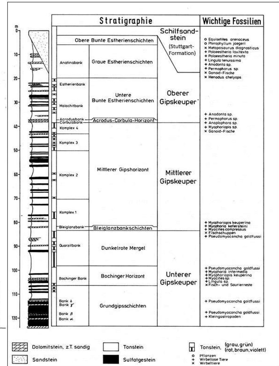
Abb. 5d: Geologisches Standardprofil des Gipskeupers (Grabfeld-Formation) - Mittlerer Keuper - im Raum Stuttgart
