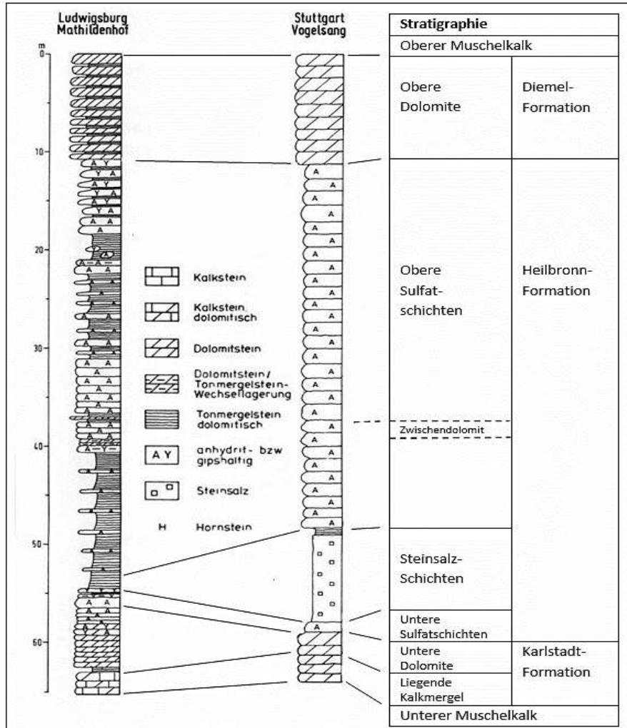
Abb. 5a: Geologische Profile des Mittleren Muschelkalks (Diemel-, Heilbronn-, Karlstadt-Formation)
