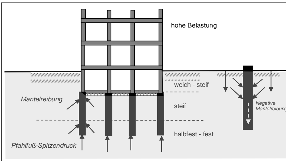
Abb. 17: Bohrpfahlgründung mit hoher Sohlpressung auf tief liegende Bodenschicht mit fester Bodenkonsistenz oder harter Festigkeit (Fels) (die Pfeile verdeutlichen die Kräfte)
