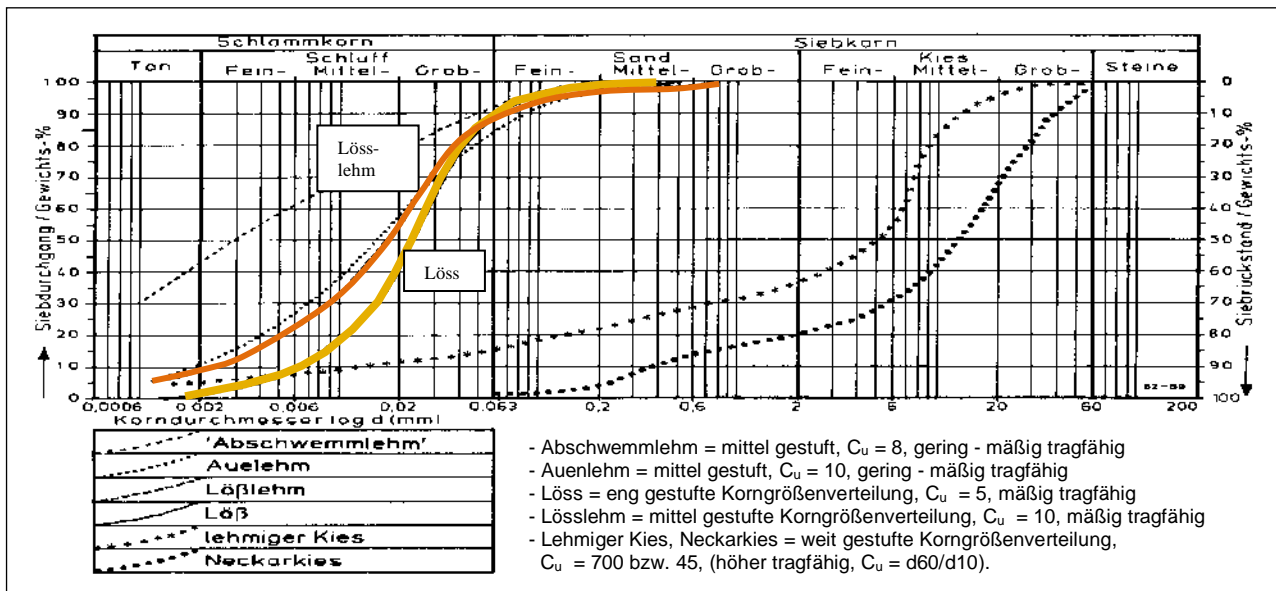
Abb.12a: Kornverteilungskurven (Kornsummenlinien, Sieblinie), Klassifikation nach DIN 4022. Das halblogarithmische Diagramm zeigt einige typische Kornverteilungskurven von Lockergesteinen im Raum Ludwigsburg. Besonders hingewiesen wird auf den unterschiedlichen Tonanteil in Lösslehm und Löss.
