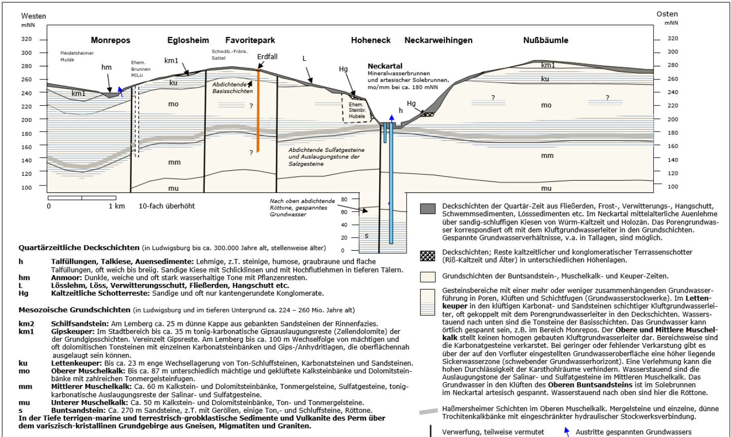
Abb. 11a: Hydrogeologischer Profilschnitt LB-Eglosheim – LB-Neckarweiningen Der Profilschnitt zeigt die drei Hauptgrundwasserstockwerke im Raum Ludwigsburg. Alle Angaben ohne Gewähr. - Oberes Stockwerk: Quartäre Deckschichten, Gipskeuper, Lettenkeuper (Porengrundwasserleiter und schichtiger Klufgrundwasserleiter, stellenweise gespannt). - Mittleres Stockwerk: Oberer Muschelkalk mit den Oberen Dolomiten des Mittleren Muschelkalks (Klufgrundwasserleiter, teilweise verkarstet), Neckarkiese (Porengrundwasserleiter). - Unteres Stockwerk: Plattensandstein im Oberen Buntsandstein (gespannter Klufgrundwasserleiter mit artesischem Austritt aus dem Bohrloch im Neckartal).
