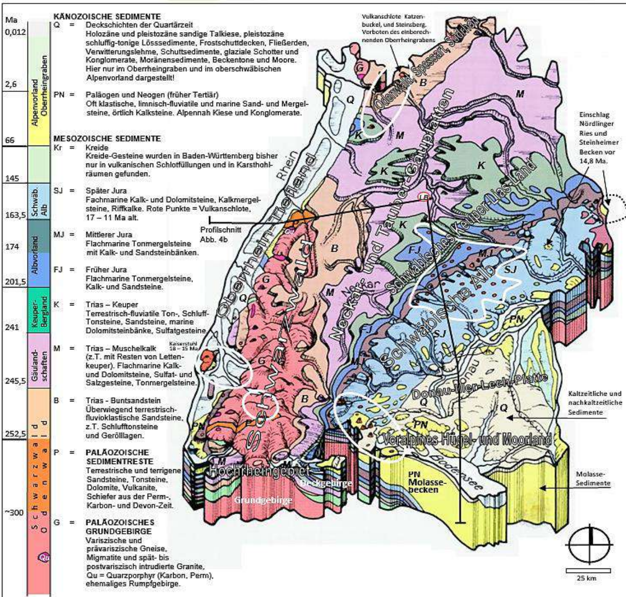
Abb. 1: Geologischer Bau von Baden-Württemberg Grafik verändert und ergänzt nach G. Wagner & A. Koch (1961), R. Hüttner und E. Villingner (LGRB-BW).
