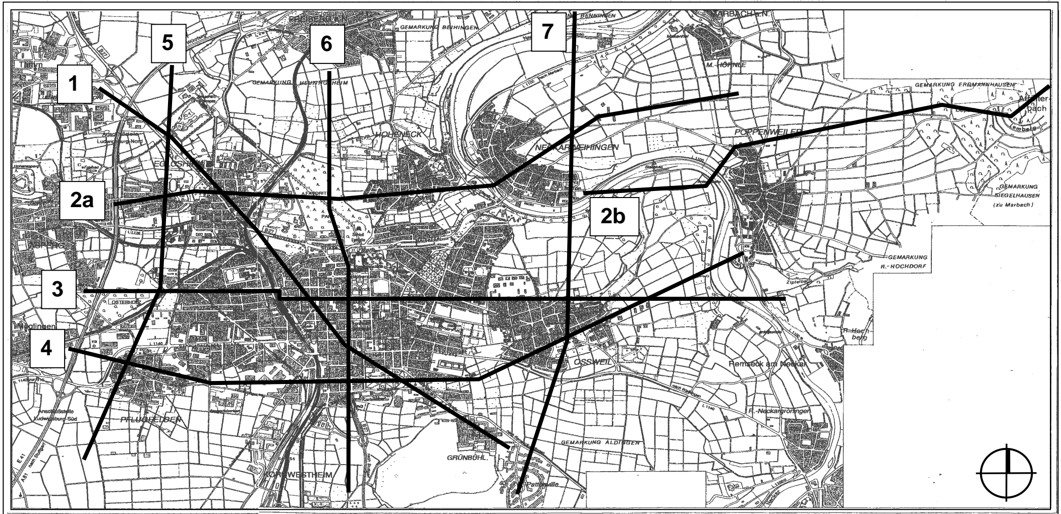
Beilage 9a: Übersicht und Lage der geologisch – hydrogeologischen Profilschnitte 1 - 7 in Ludwigsburg. Alle Angaben ohne Gewähr.
