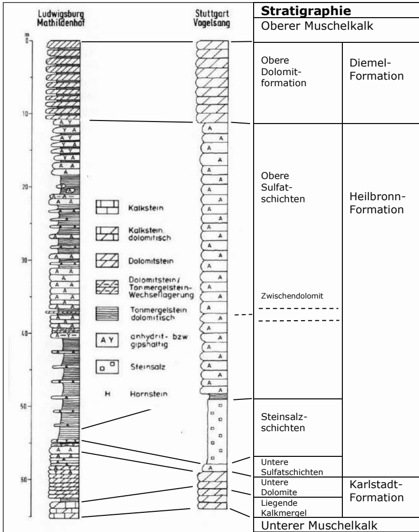
Abb. 5a: Geologische Profile des Mittleren Muschelkalks aus Tiefbohrungen (Diemel-, Heilbronn- und Karstadt-Formation). Links: Mittlerer Muschelkalk in der Grundwasserbohrung Mathildenhof in Ludwigsburg mit ausgelaugten Steinsalzschiefer und Sulfatschichten in fortschreitender Auslaugung. Rechts zum Vergleich: Mittlerer Muschelkalk in Stuttgart mit vollständiger Sulfat- und Salinarformation. Schichtprofile ergänzt aus: H. Brunner (1998): Geologische Karte von Baden-Württemberg 1 : 50 000, Erläuterungen Stuttgart und Umgebung. LGRB-BW, Freiburg.
