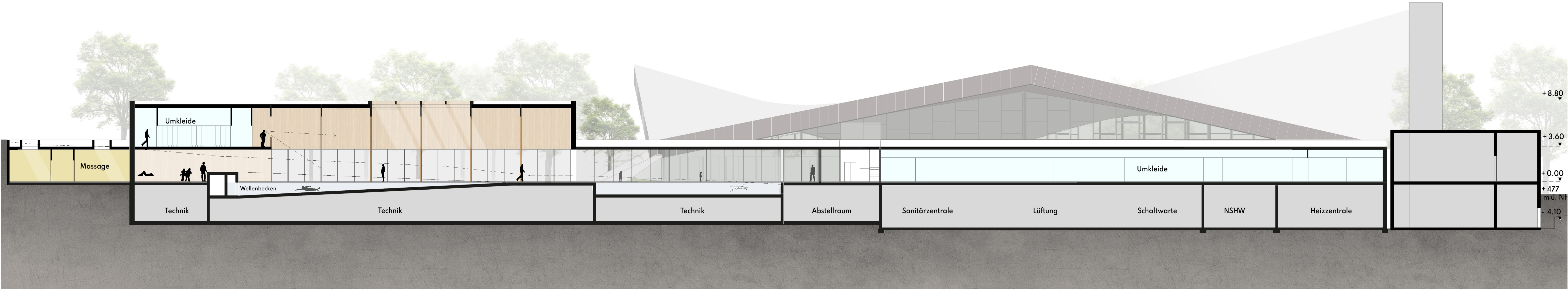
Schnitt A-A 1:200
