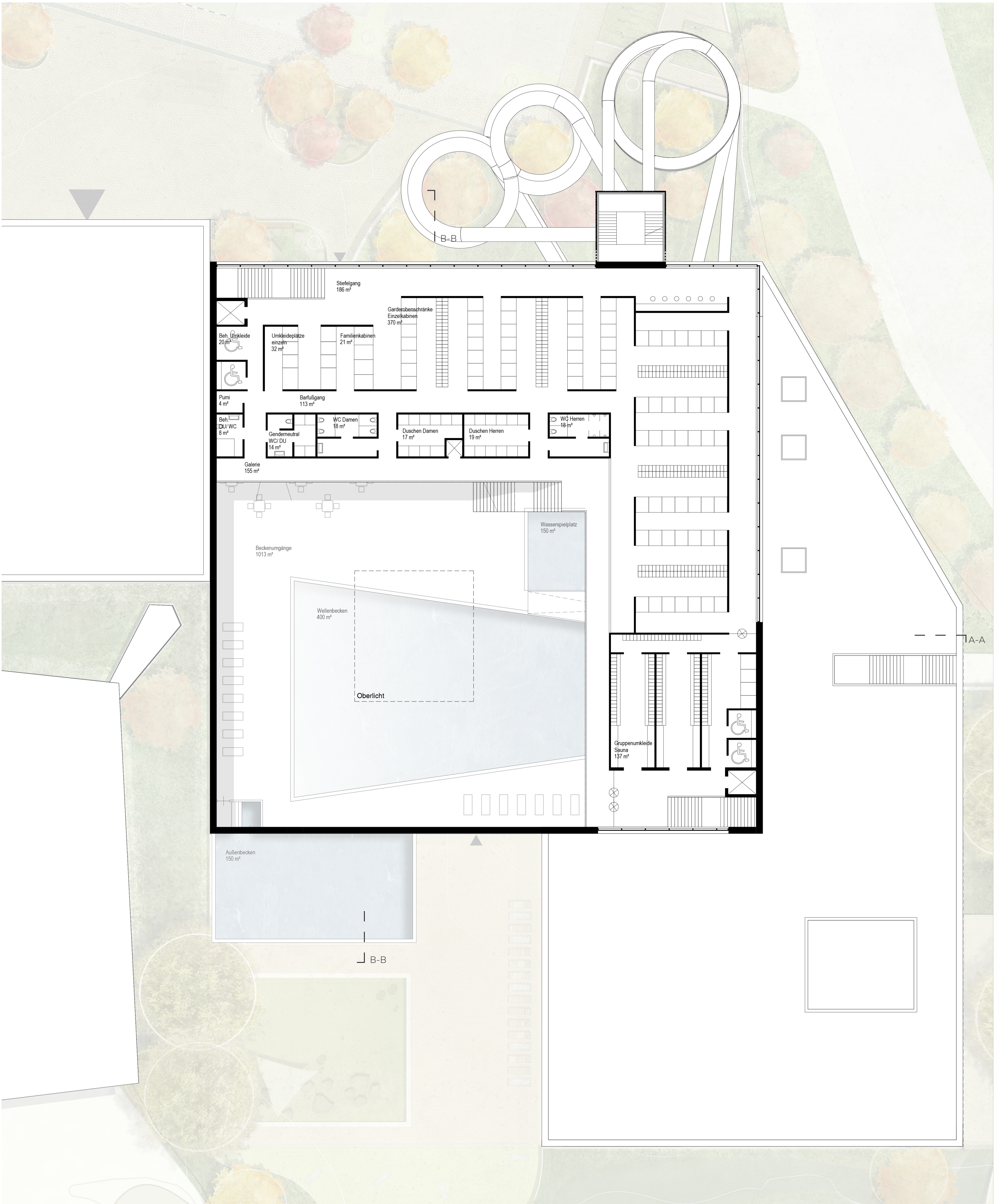
Grundriss 1.OG 1:200
