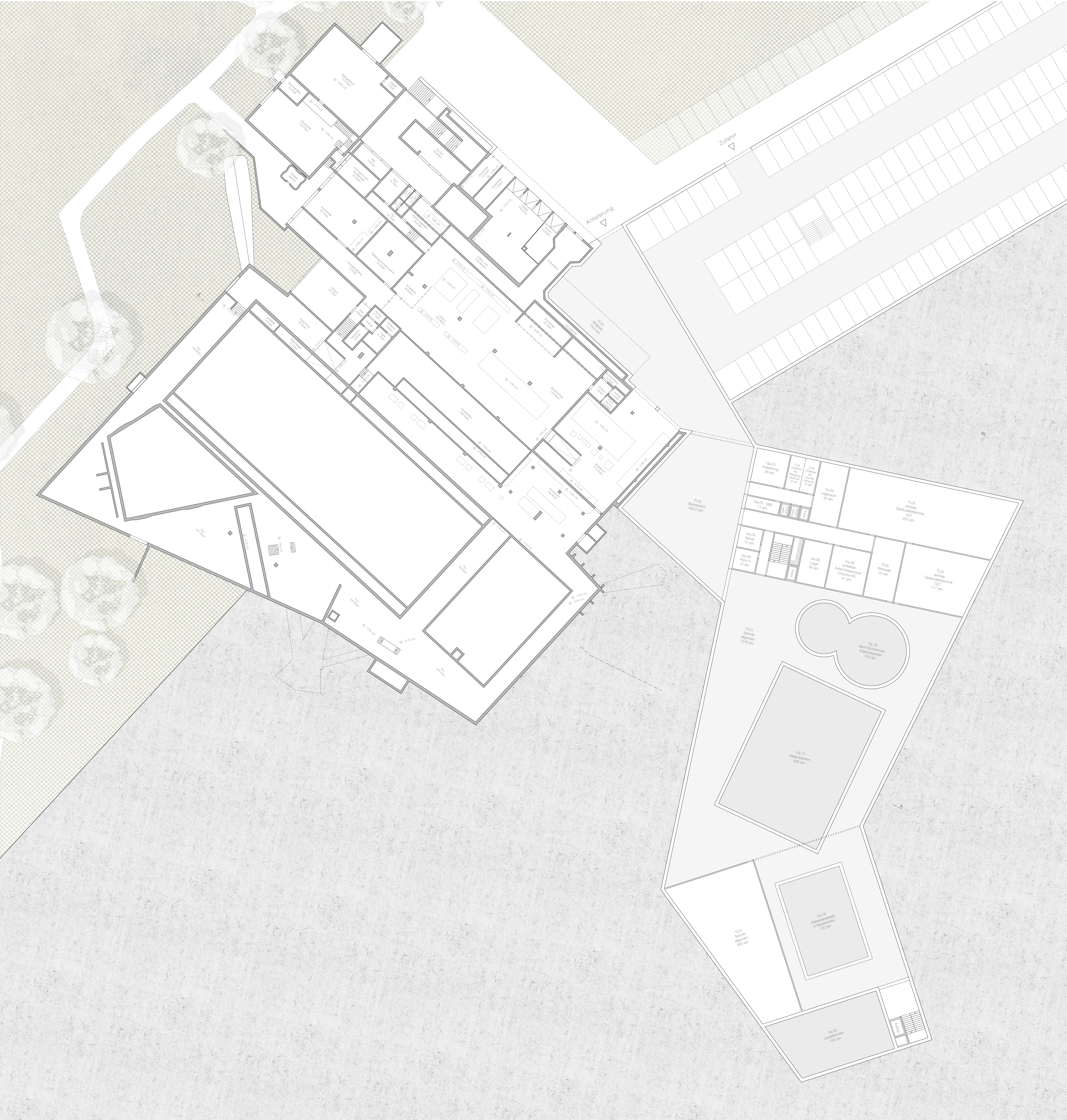
Grundriss Untergeschoss 1:200
