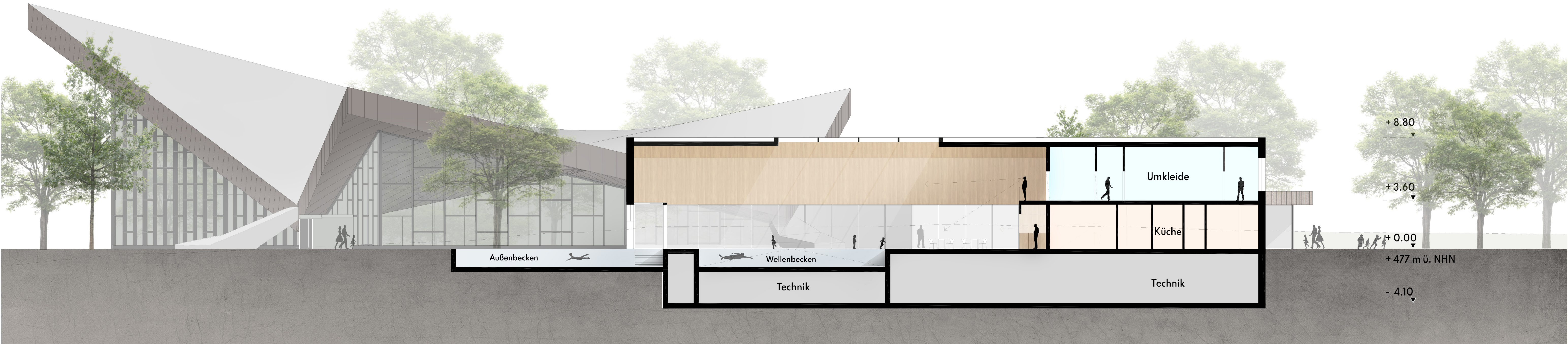
Schnitt B-B 1:200
